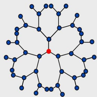
Dendrimer 15 - 200 nm
