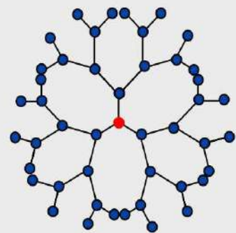
Dendrimer 15 - 200 nm
