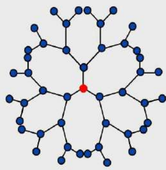
Dendrimer 15 - 200 nm
